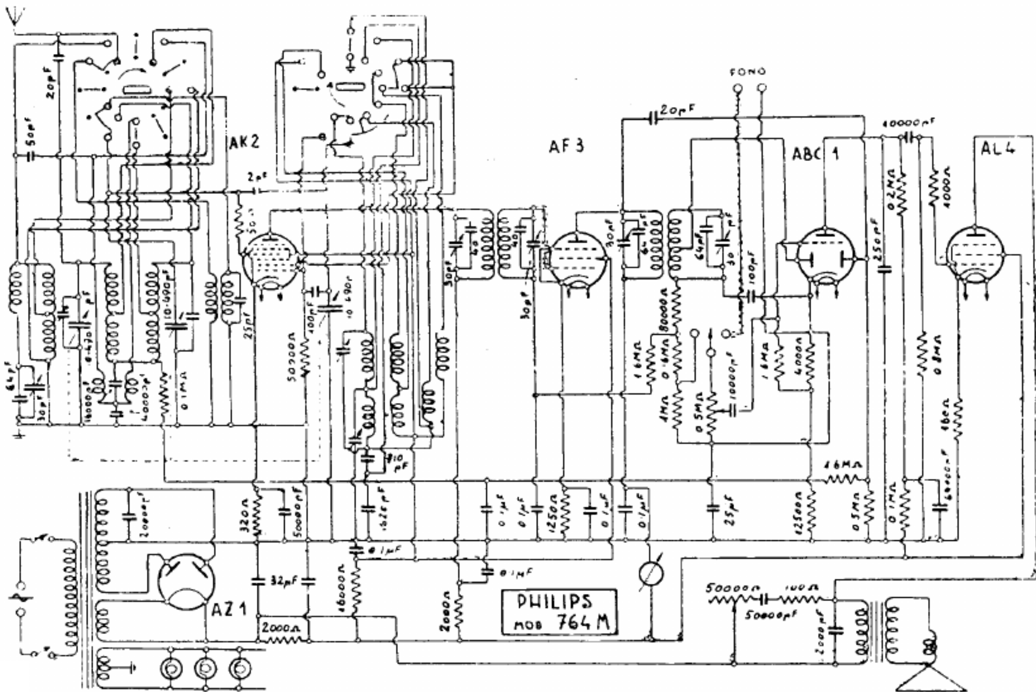
PHILIPS RADIO — Modello « 764 M » Produzione 1937. Media frequenza: 128 kHz
